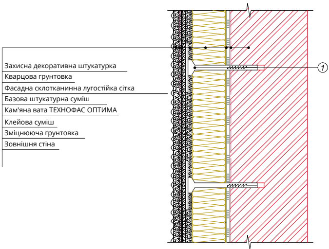
① Тарілчастий дюбель з розпірним елементом
